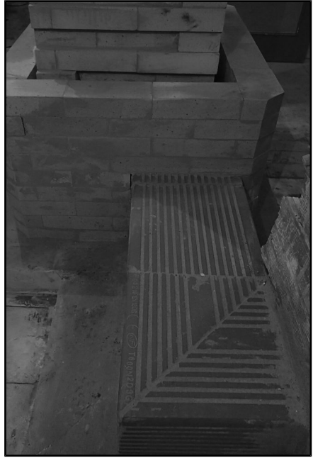
Connexion du poêle au conduit sans et avec banc
